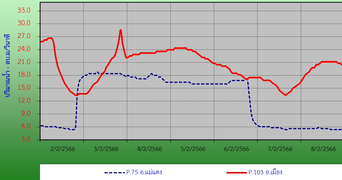
กราฟแสดงปริมาณน้ำปิงรายชั่วโมงรอบวันที่ 5/2566 ที่สถานีแม่ น้ำปิง ( P.75) บ้านซ้อแล อ.แม่แตง และที่สถานีแม่ น้ำปิง (P.103) บ้านป่าซ่อยใต้ อ.เมือง จ.เชียงใหม่
